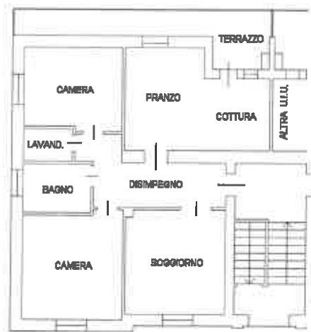
PIANO RIALZATO - H=3,00 m
